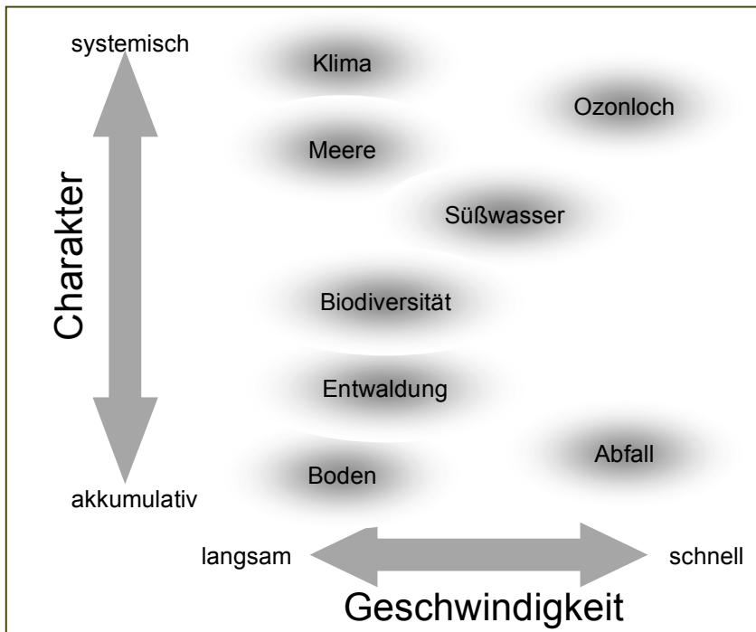
Abb.7: Charakter und Geschwindigkeit verschiedener globaler Umweltprobleme
